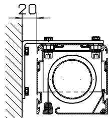
Wandhalterung direkte Montage
